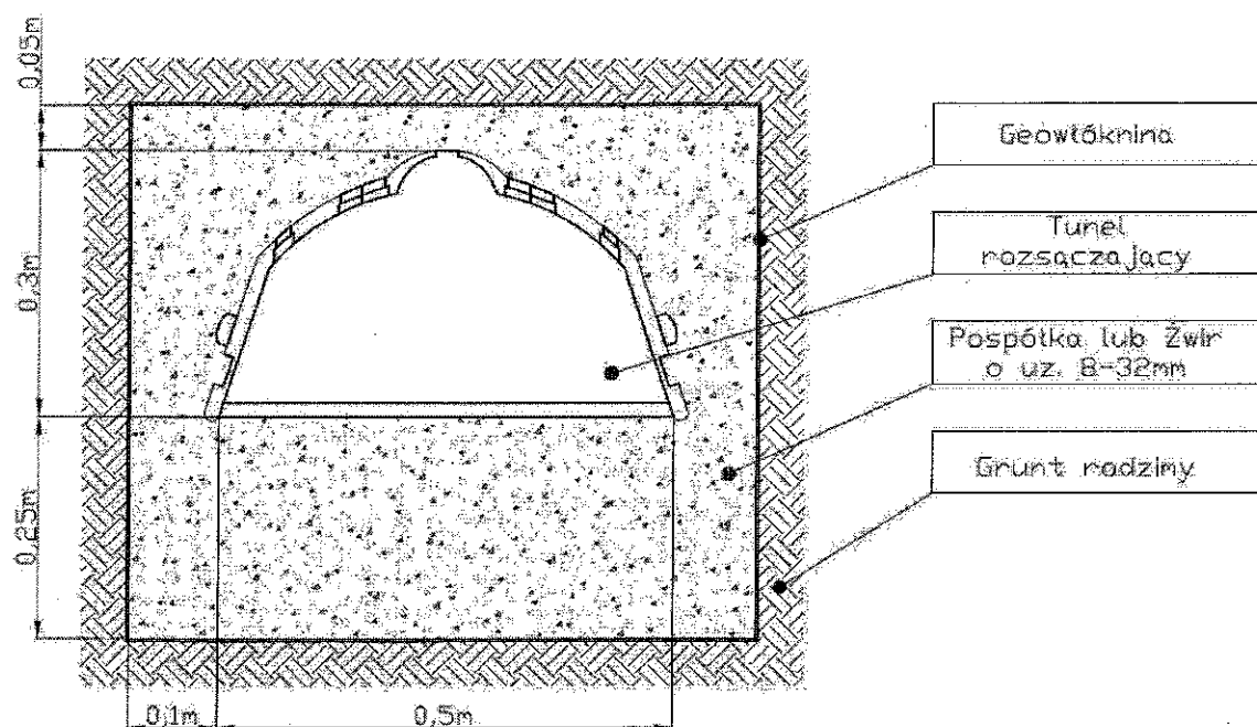
Ryc. 1. Schemat montażu tunelu.
